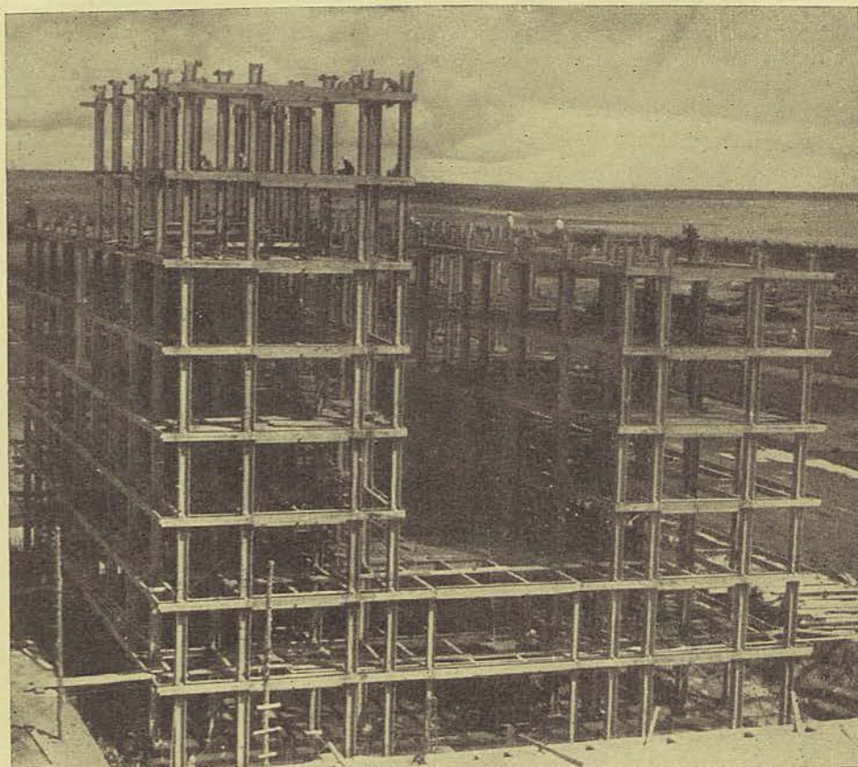
1. Cúpula do Senado Federal pronta para receber o concreto. 2. Plenário da Câmara dos Deputados. 3. O edifício anexo ao Congresso Nacional com a estrutura metálica em andamento.
