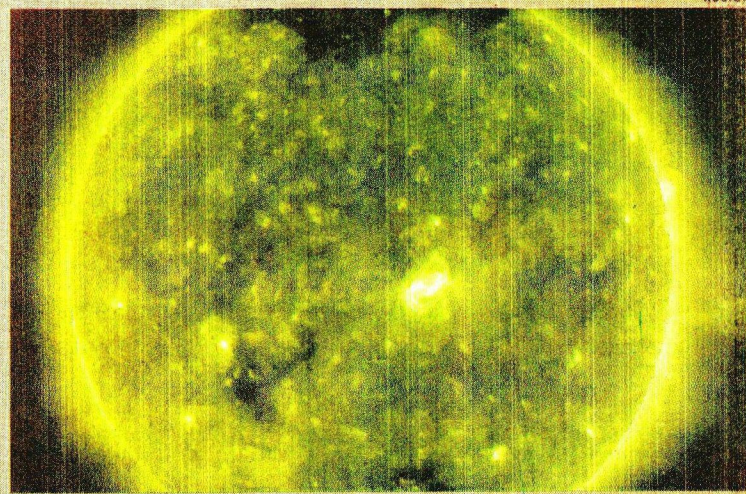
O SOL DE PERTO — O diretor da Agência Espacial Européia, Roger Bonnet, mostra imagem do Telescópio de Imagens Ultravioletas Extremas, a bordo do Observatório Solar e Heliosférico (SOHO). A atmosfera externa do Sol revela violentas erupções, a 1.500.000 °C.
